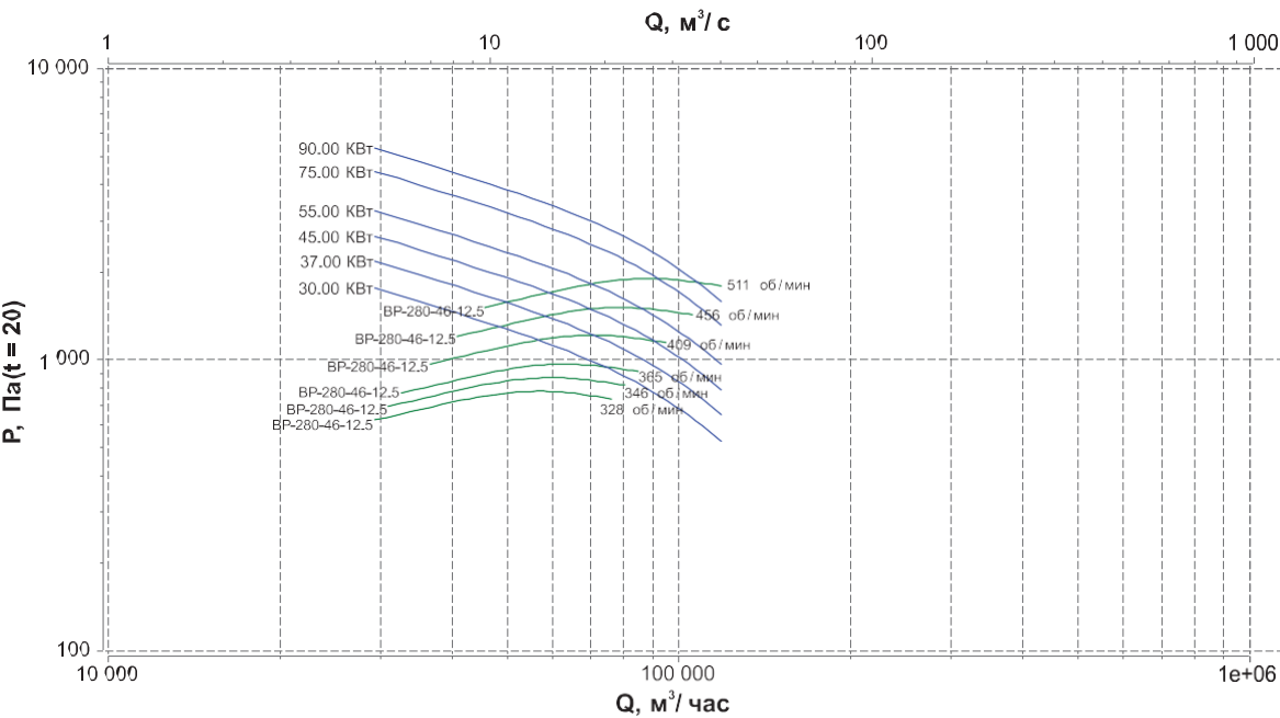
BP 280-46-12,5 схема 5
