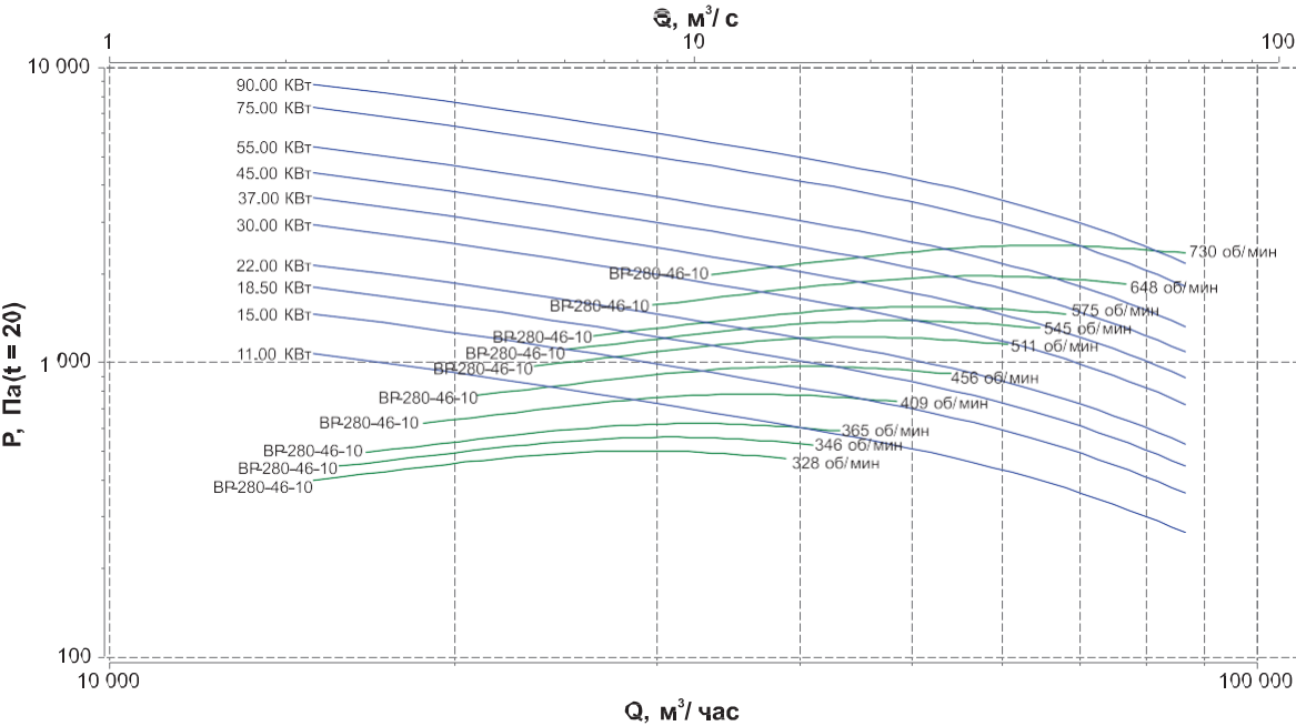
BP 280-46-10 схема 5
